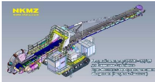
Kompaktschaufelradbagger ER1500-9,5/0,5 (nkmz)
